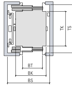
Double accès Porte télescopique
